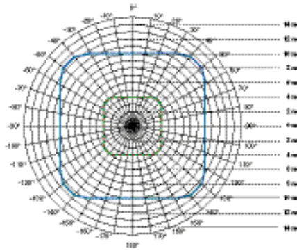
Presence Control PRO IR Quattro HD, монтажна височина 2,80 м син = тангенциално, червен = радиално, зелен = присъствие
